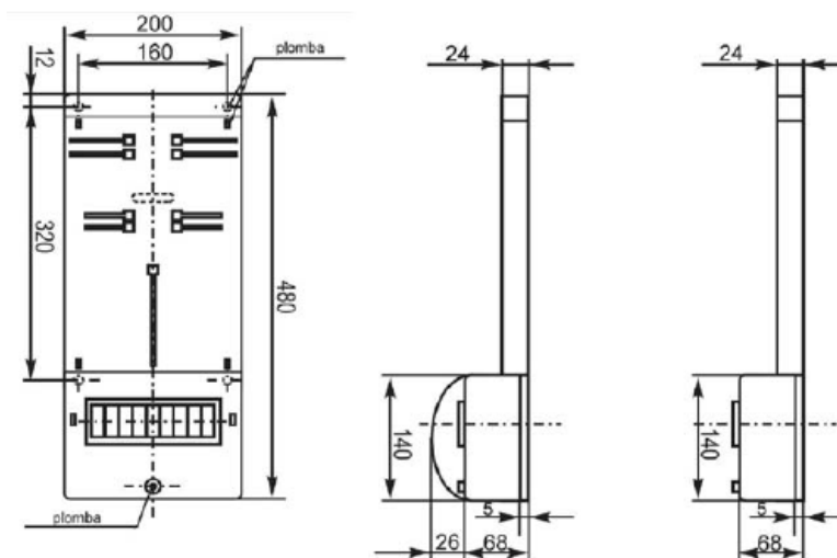
KÖRVONALRAJZ:
